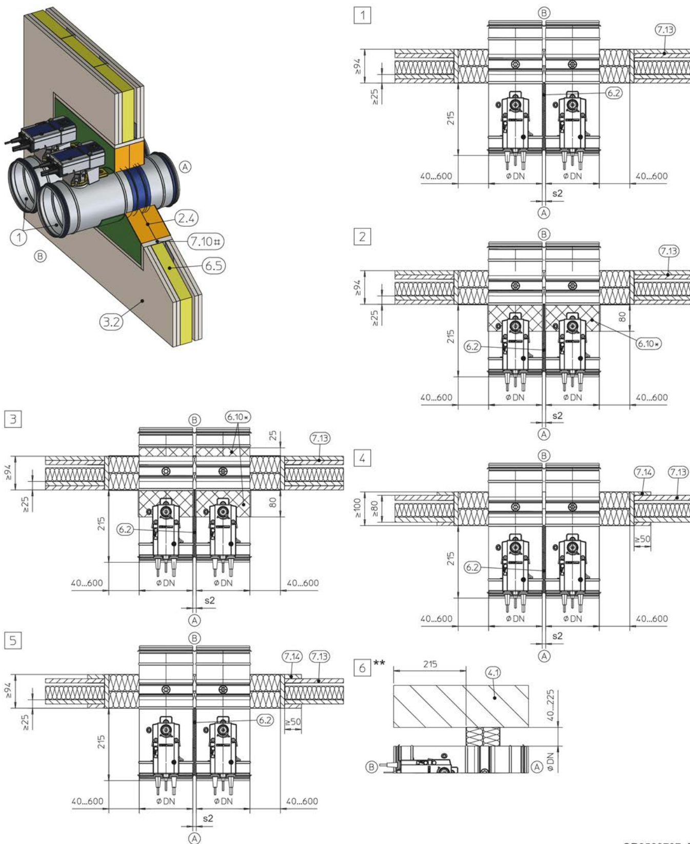
Fig. 70: Installazione a secco in una parete divisoria leggera, con isolante antincendio, 'affiancata', l'illustrazione mostra l'installazione fianco a fianco (si applica inoltre alle installazioni di serrande una sopra l'altra)
