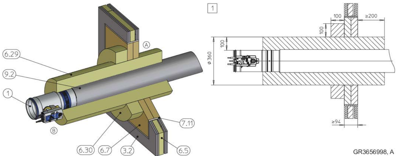
Fig. 66: Installazione a secco senza malta lontano da una parete divisoria leggera, con isolante antincendio
