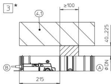
Fig. 90: Installazione a base di malta in una parete piena in legno o in legno lamellare a strati incrociati, 'affiancata', l'illustrazione mostra l'installazione fianco a fianco (si applica inoltre alle installazioni di serrande una sopra l'altra)
