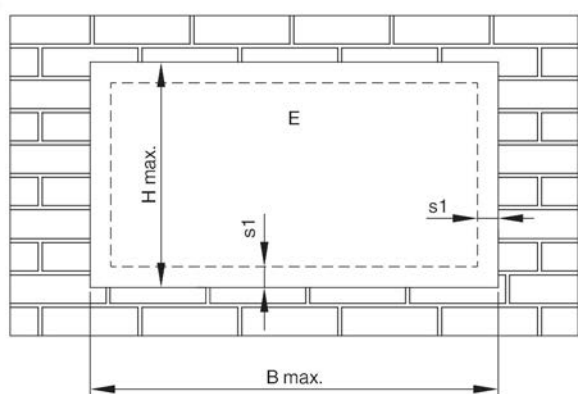
Fig. 17: isolante antincendio – installazione in una parete solida, parete divisoria leggera o parete con intelaiatura di legno
