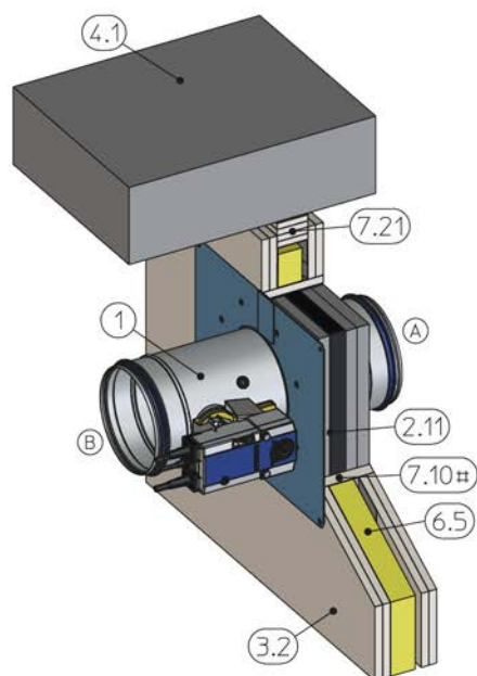
Fig. 60: Installazione a secco senza malta con kit di installazione TQ / TQ2 in una parete divisoria leggera, sotto al collegamento flessibile al soffitto
