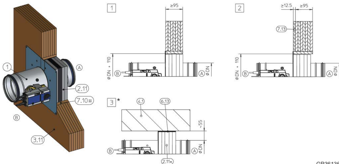
Fig. 91: Installazione a secco senza malta in una parete piena in legno o in legno lamellare a strati incrociati, con kit di installazione TQ / TQ2
