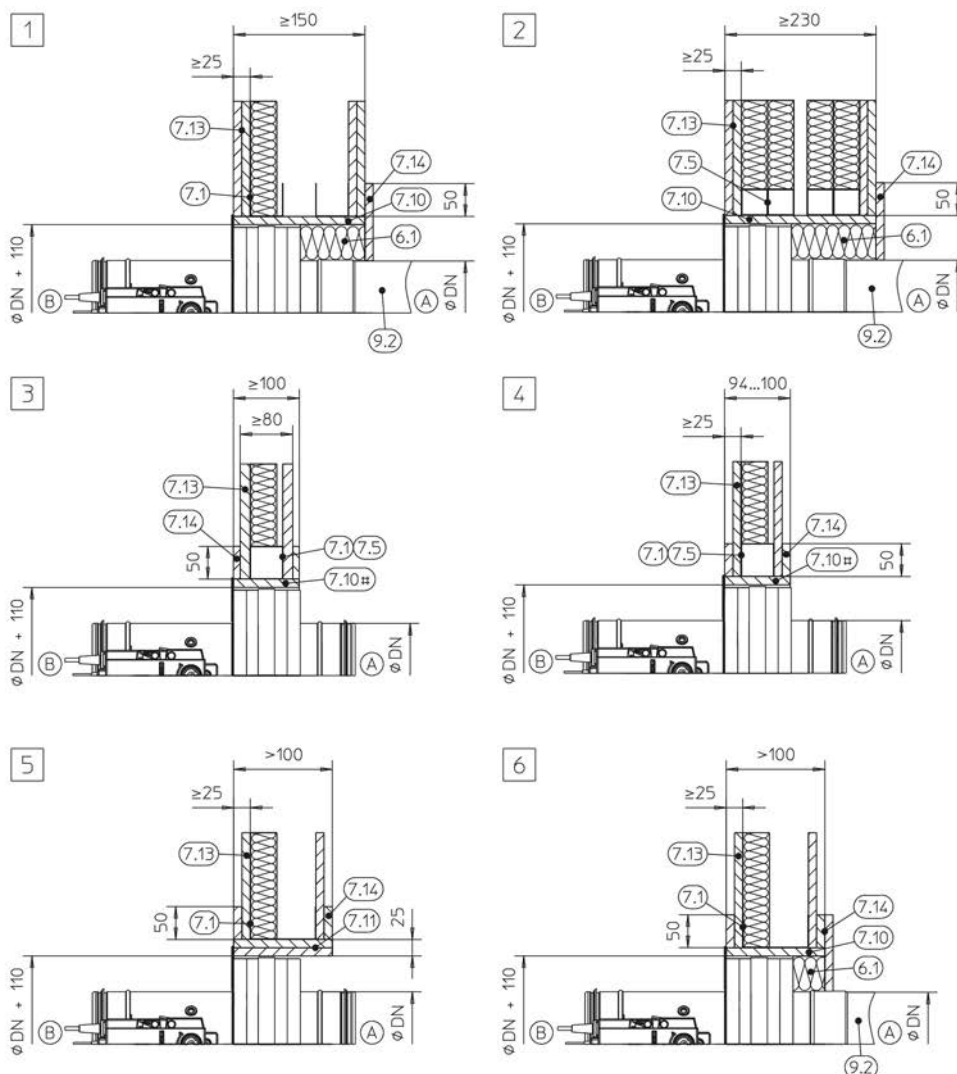
Fig. 58: Installazione a secco senza malta in una parete divisoria leggera, con kit di installazione TQ / TQ2
