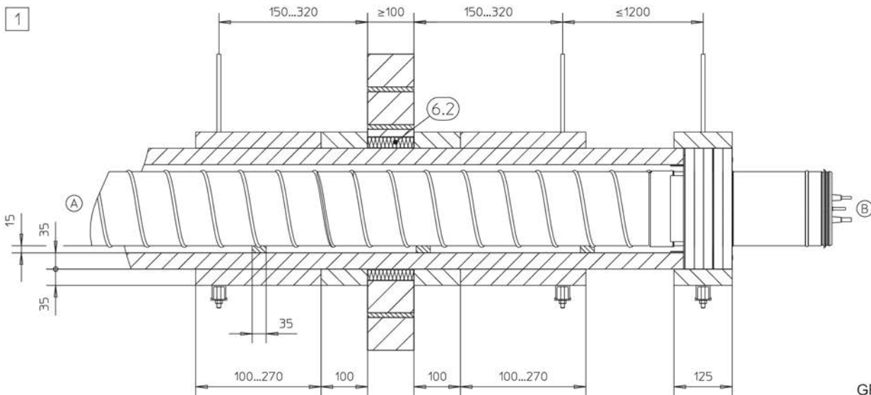
Fig. 43: Installazione a secco senza malta lontano da una parete piena con attraversamento della parete, rivestimento su tre lati
